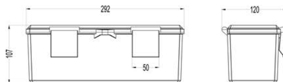
0001.4002.XXX - TOOL BOX MINI SIZE
